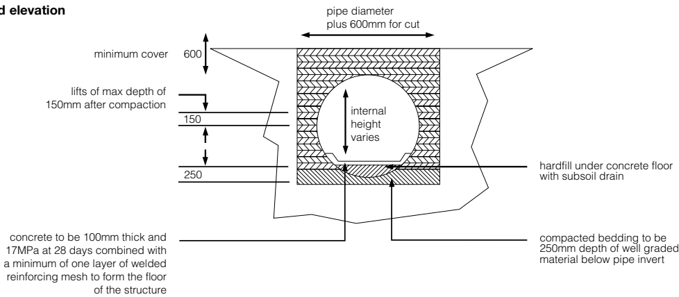
end elevation
