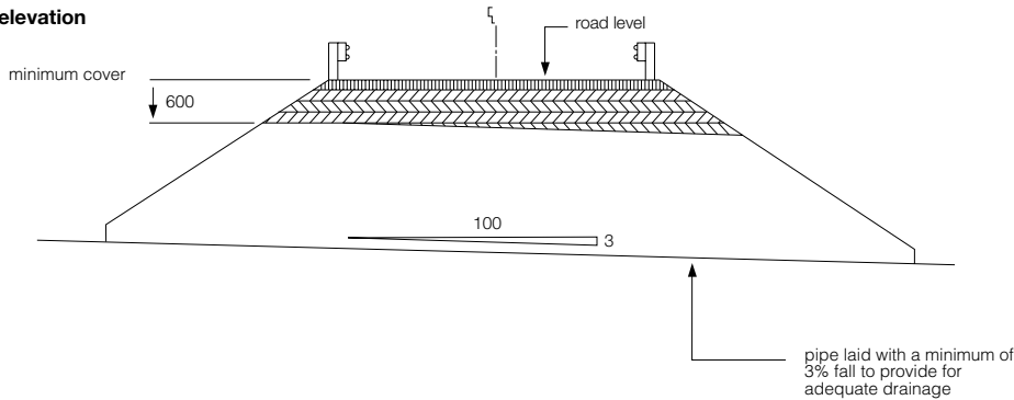
end elevation
