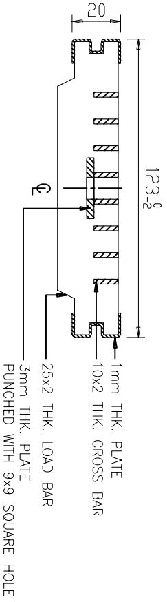
SECTION A-A
